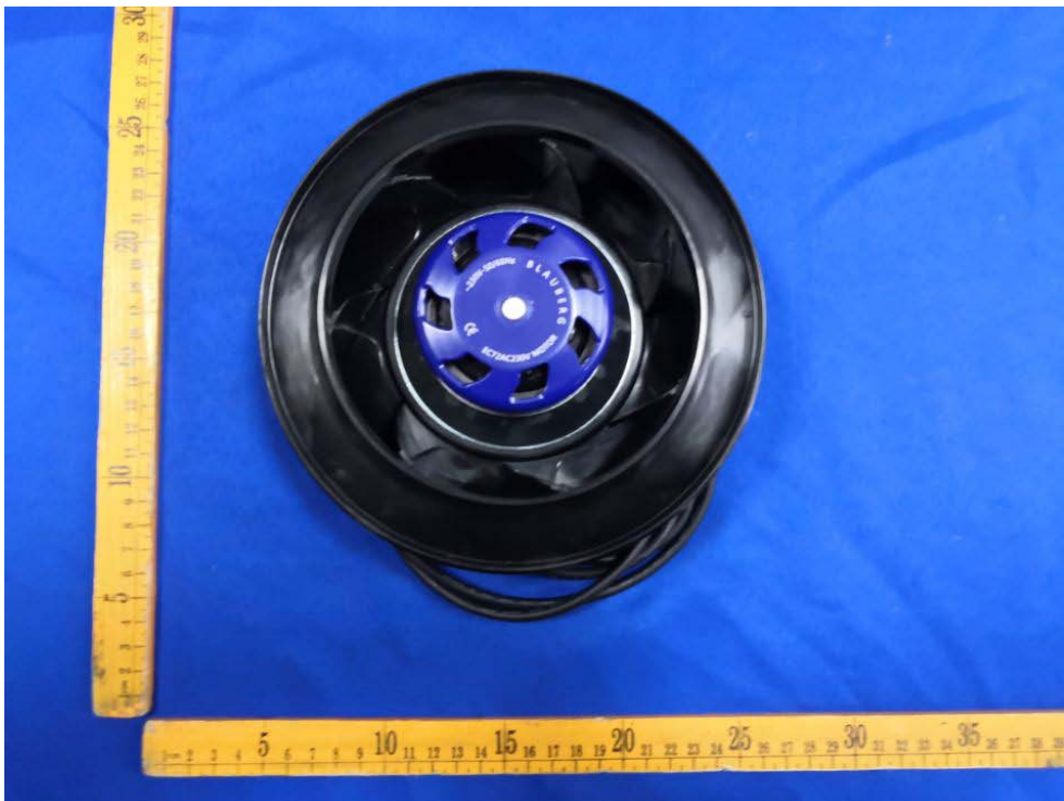
Test sample-IP5X
