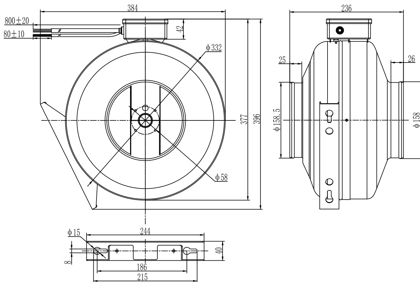
支架安装孔位图
