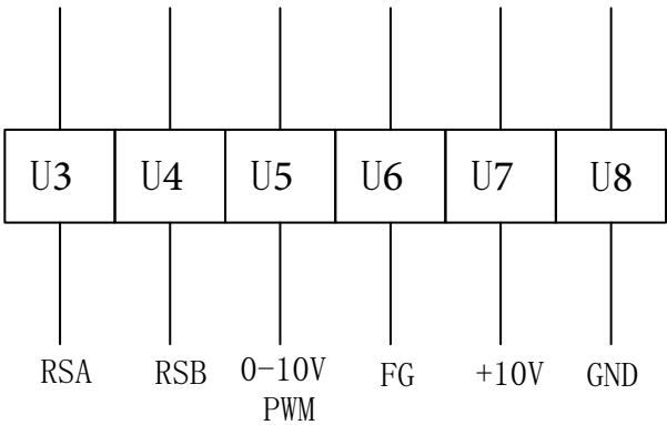
控制线
