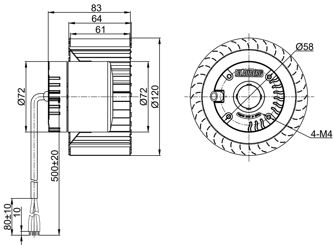
外形图
