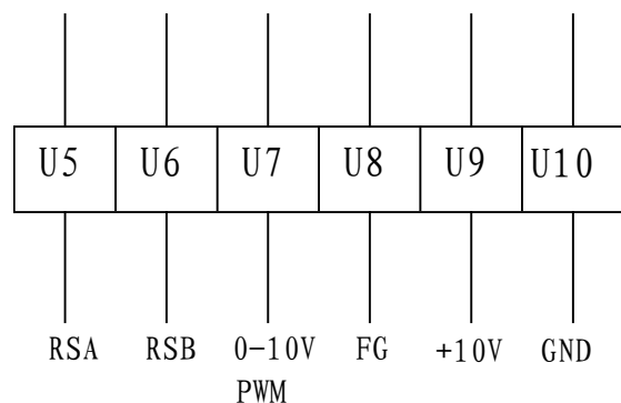
控制线
