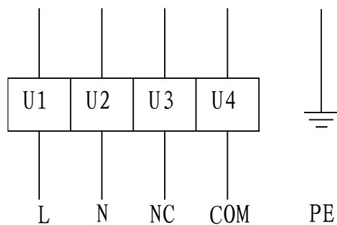
电源线
