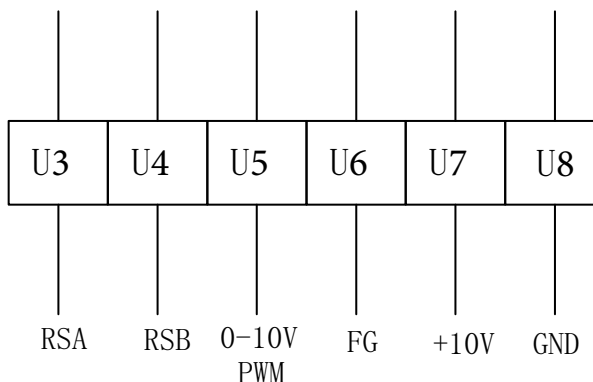
控制线
