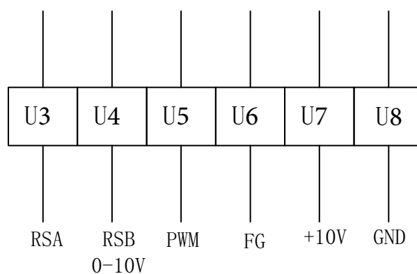
控制线
