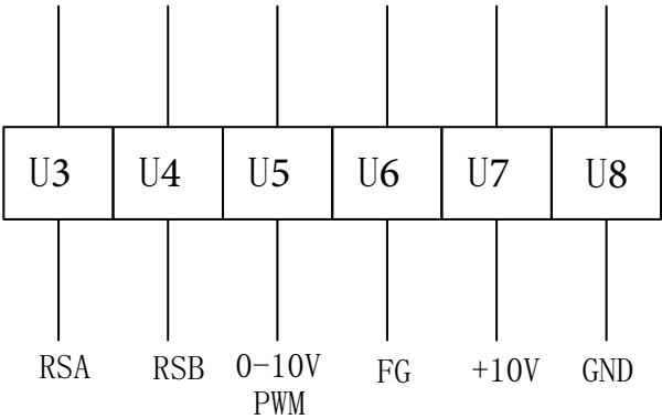
控制线
