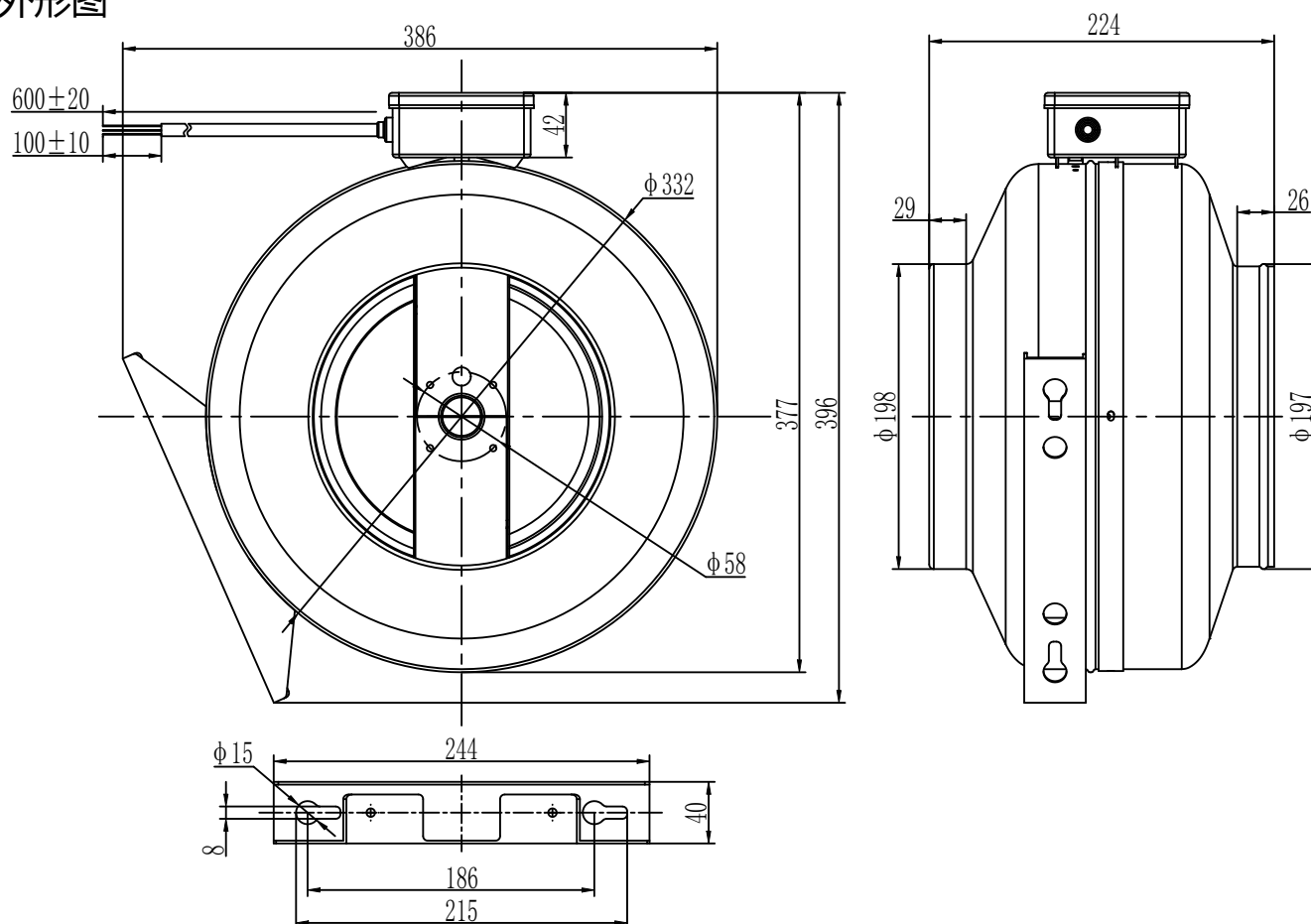
支架安装孔位图
