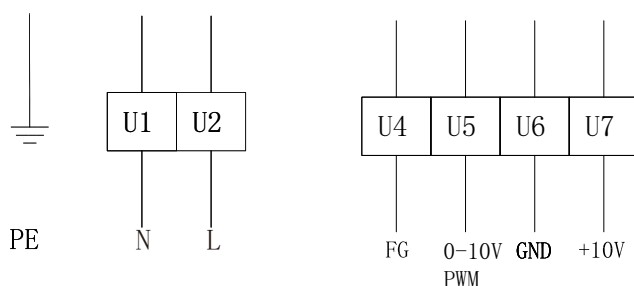
控制线
